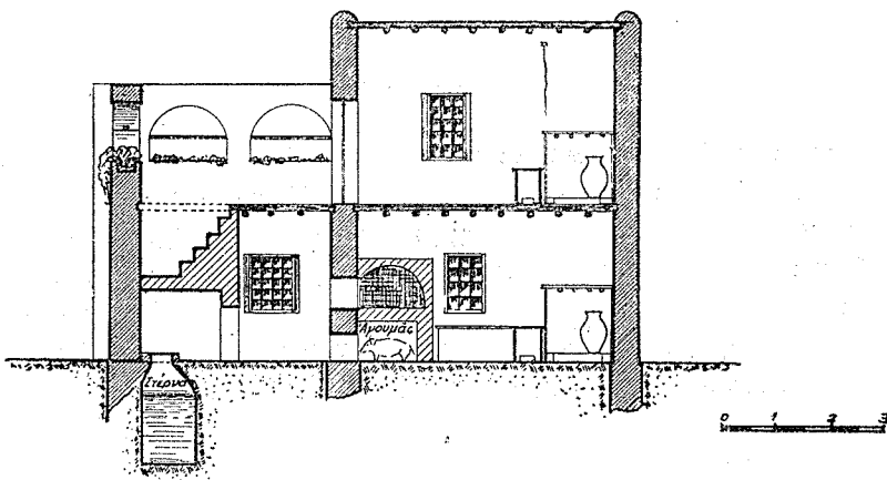
Τομή τοῦ σπιτιοῦ τῆς Ἄννας Ζαγράφου στὸ Ἐμπορεῖο. (Ἀπὸ τὸ βιβλ. «Δωδεκάνησος» τοῦ Ὑπουργείου Ἀνοικοδομήσεως).
