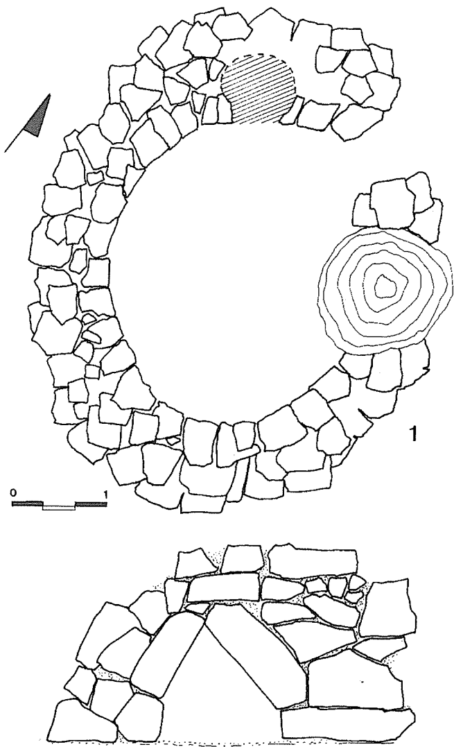
Σχέδ. 3. Το «τυροζόμι» 1.
