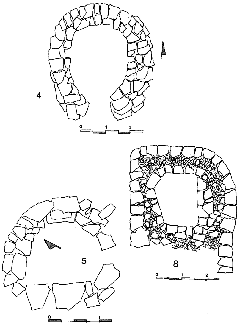
Σχέδ. 6. Πεταλοειδή και τετράπλευρα κτίσματα.
