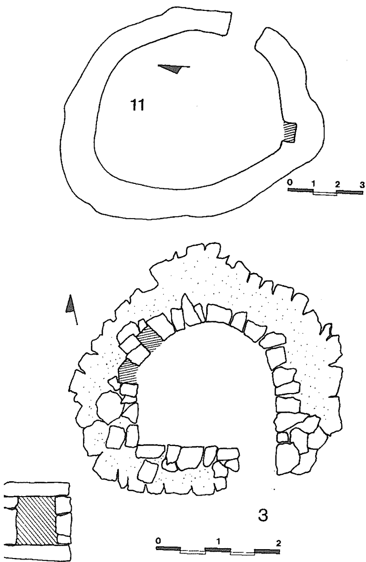
Σχέδ. 5. Κατοικία βοσκού (II) και «τυροκόμι» (3).
