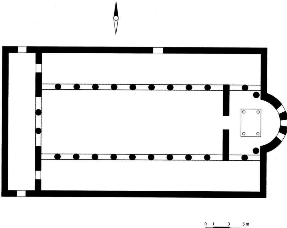
Κάτοψη της Βασιλικής του Αρχ. Μηχ. Δρ. Ανδ. Θεοδοσίου, σύμφωνα με τις μετρήσεις Ι. Βολανάκη
