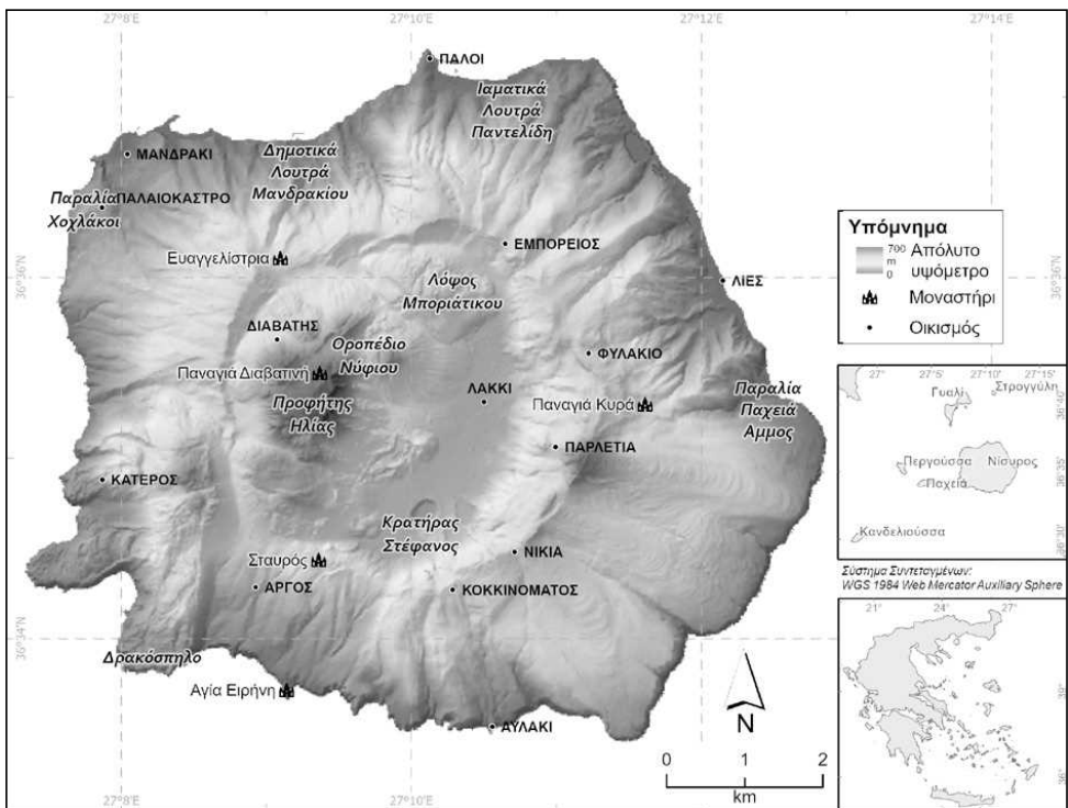
Εικόνα 2. Ψηφιακό υψομετρικό μοντέλο (DEM) του ηφαιστειακού νησιού της Νισύρου με τις σημαντικότερες τοποθεσίες.
