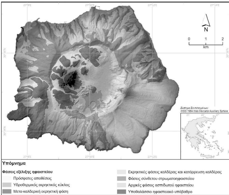
Εικόνα 3. Οι εκρηκτικοί κύκλοι του ηφαιστειογενούς νησιού της Νισύρου.
