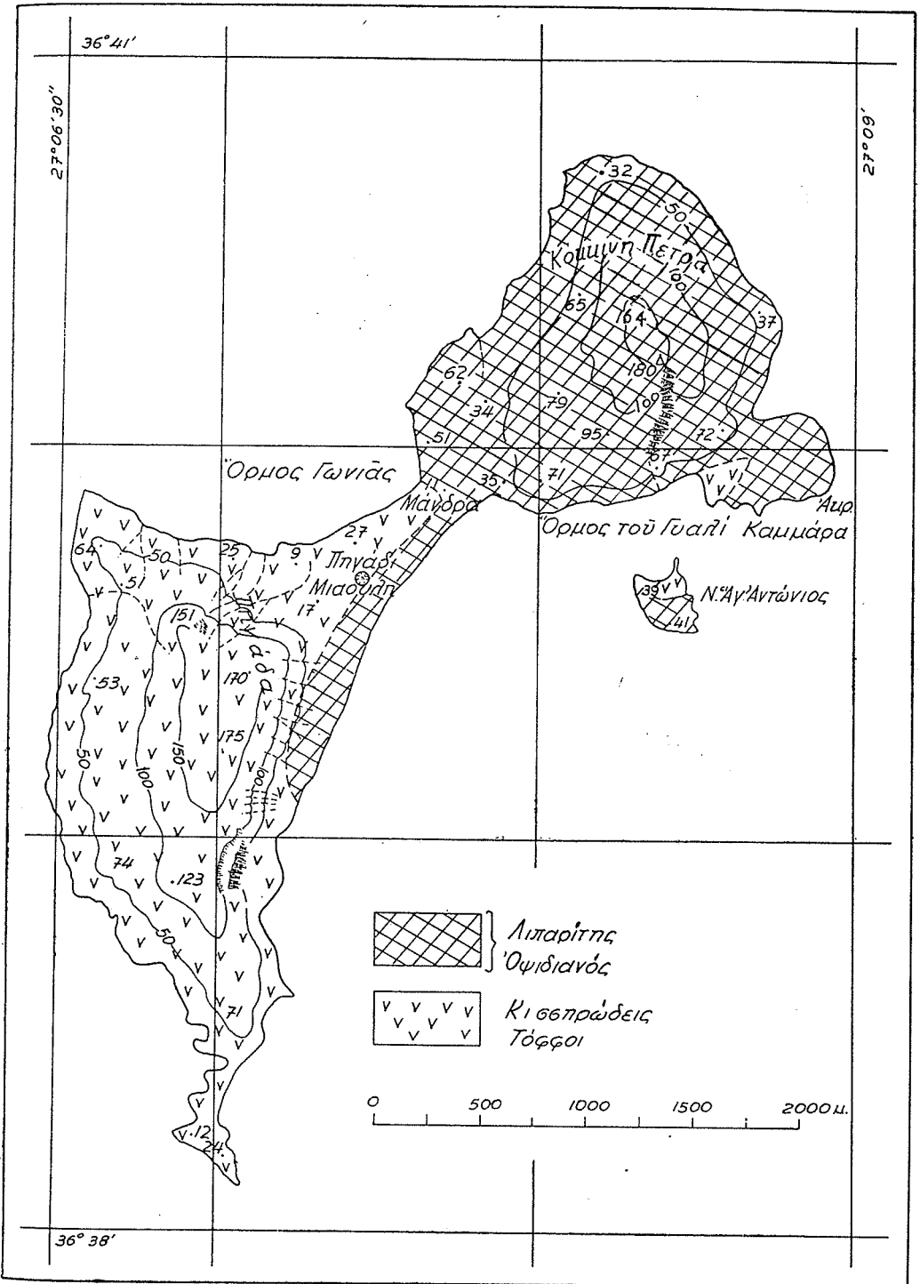
Σχ. 2.— Γεωλογικός χάρτης της νησίδος Γουαλί (κατά τὸν Α. Μαρτελλί).
