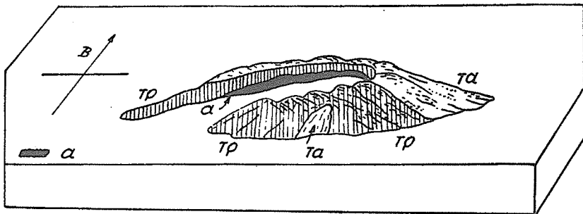
Σχ. 5— Τὰ πρῶτα στάδια ἐξελιξέως τοῦ ἡφαιστείου. α = ἀνδεσίται. τα = τραχυανδεσίται, τρ = τραχεΐται.
