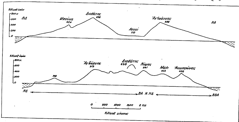
Σχ. 1: Δύο τομαὶ διὰ μέσου τῆς Νισύρου.
