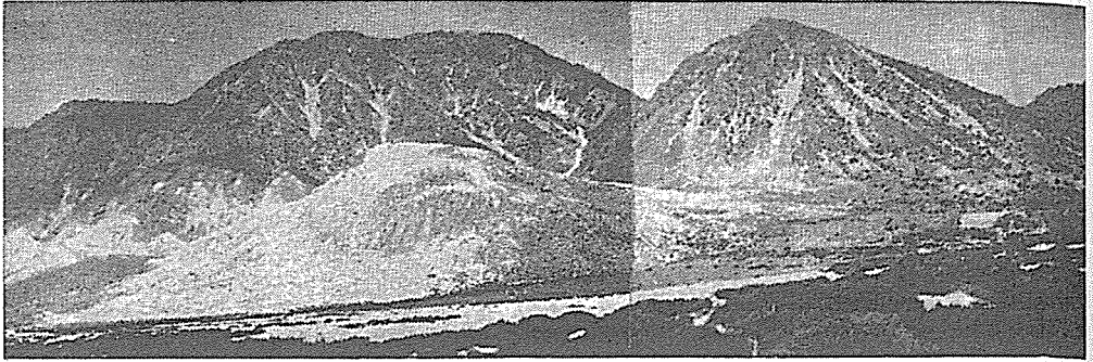
Σχ. 7.— Οἱ δύο ἠφαιστειοὶ θόλοι, ὁ Πρόφ. Ἡλίας (Διαβάτης) ἀριστερὰ καὶ ὁ Νύφιος δεξιὰ. Ἐμπροσθεν τοῦ Πρόφ. Ἡλίας ὁ λόφος 211. Διακρίνεται ἐπὶ τῆς κορυφῆς τοῦ Πρόφ. Ἡλίας τὸ ἐγκατακρημνισιγενὲς κρατηροειδὲς κοίλωμα.
