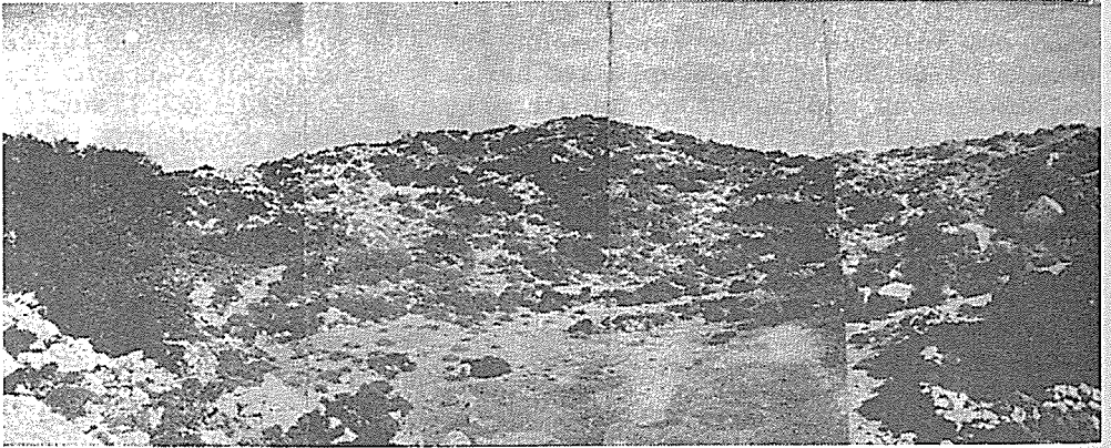
Σχ. 8.— Τὸ ἐγκατακρημνισιγενὲς κρατηροειδὲς κοίλωμα ἐπὶ τῆς κορυφῆς τοῦ ἠφαιστείου θόλου τοῦ Πρόφ. Ἡλίας (Διαβάτη).
