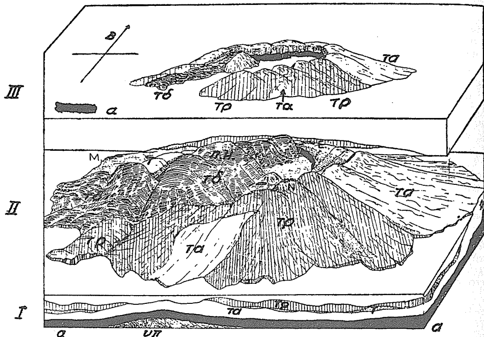
Σχ. 4.— Τὰ στάδια ἐξελίξεως τοῦ ἥφαιστείου τῆς Νισύρου (κατὰ τὸν Α. DESIO). Μ=Μανδράκι. Ε = Ἐμπορειός. Ν = Νικιά. Π.Η = Προφήτης Ἡλίας. α = ἀνδεσίται. τα = τραχουανδεσίται. τρ = τραχεΐται. τδ=τραχειδακίται. Τὰ διὰ στιγμῶν σημειούμενα τμήματα εἶναι οἱ τόφφοι. ὑπ=τὸ ἐκ μὴ ἥφαιστειογενῶν πετρωμάτων ὑπόβαθρον τῆς νήσου.
